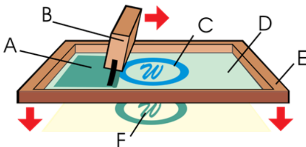
A encre - B porte raclette + raclette - C motif à imprimer - D écran = toile + film - E cadre - F image imprimée.
